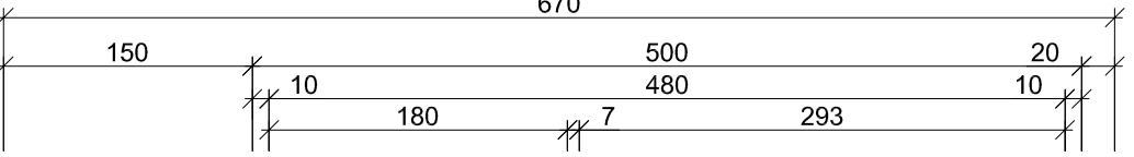
Ansicht B
